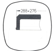
Br 288 x 245 / 276 x 230 Talon Konkav
