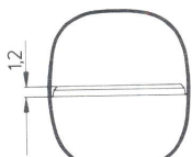
Pl. Br 195_{/160} \times 174_{/130}
